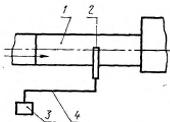
1—измерительный патрубок; 2—термоанемометр; 3—электродоизмерительный прибор; 4—соединительные провода
