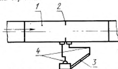
1—измерительный трубопровод; 2—диафрагма или сопло; 3—измерительный прибор (микрометр, U-образный манометр); 4—соединительные шланги.
