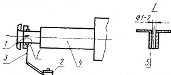
1—измерительный коллектор; 2—измерительный прибор (микроанемометр, С-образный манометр); 3—соединительные шланги; 4—патрубок; 5—приемник давления.
