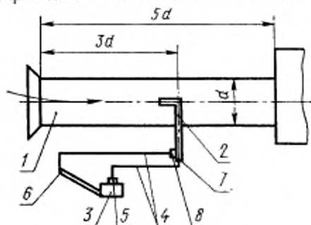
1—измерительный патрубок; 2—трубка Прандтля; 3—измерительный прибор (микроанометр, U-образный манометр); 4—соединительные шланги; 5—штуцер большого давления; 6—штуцер меньшего давления; 7—штуцер полного давления; 8—штуцер статического давления.
