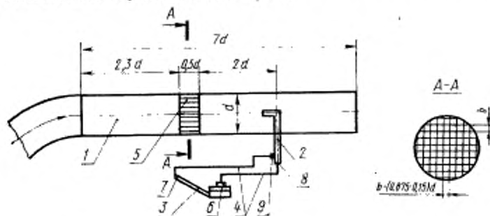
1—измерительный патрубок; 2—трубка Прандтля; 3—измерительный прибор (микроанометр, U-образный манометр); 4—соединительные шланги; 5—прямая решетка; 6—штуцер большого давления; 7—штуцер меньшего давления; 8—штуцер полного давления; 9—штуцер статического давления.
