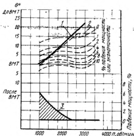
1 дотонационная характеристика заданного бензина; 2 выбранная характеристика автомата; 3 потери мощности
