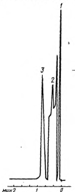
Типовая хроматограмма технического дифенила, полученная при 180^{\circ}\text{C}
