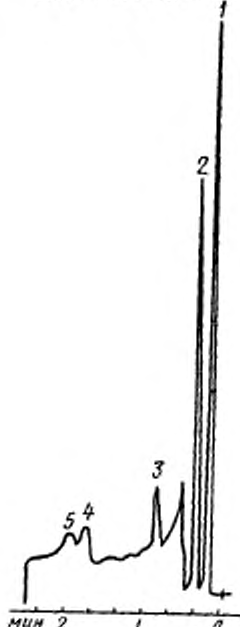
Типовая хроматограмма технического дифенила, полученная при 240^{\circ}\text{C}
