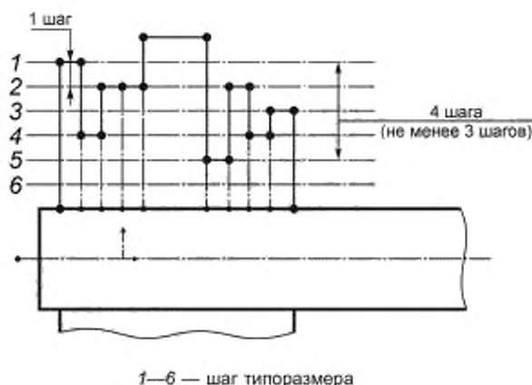
Рисунок 2 — Схема перепада между максимальным и минимальным значениями кода
