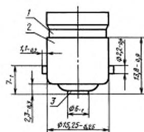
Цоколь типа P15s/14
