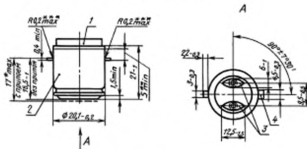
Цоколь типа P20d/21
