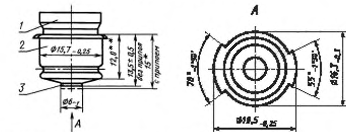
Цоколь типа P19s/13
