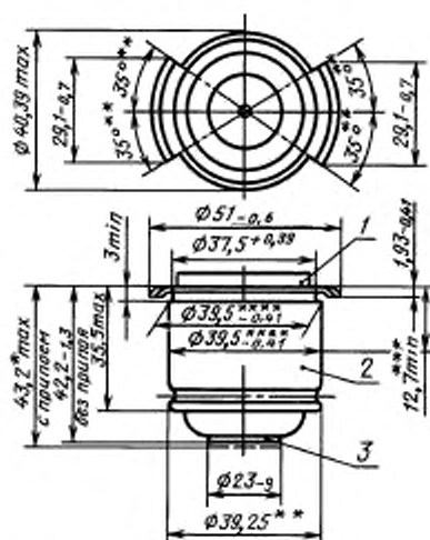
Цоколь типа P40s/41
