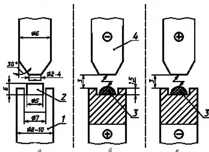
Расположение электродов с пробями при съемке спектрограмм
