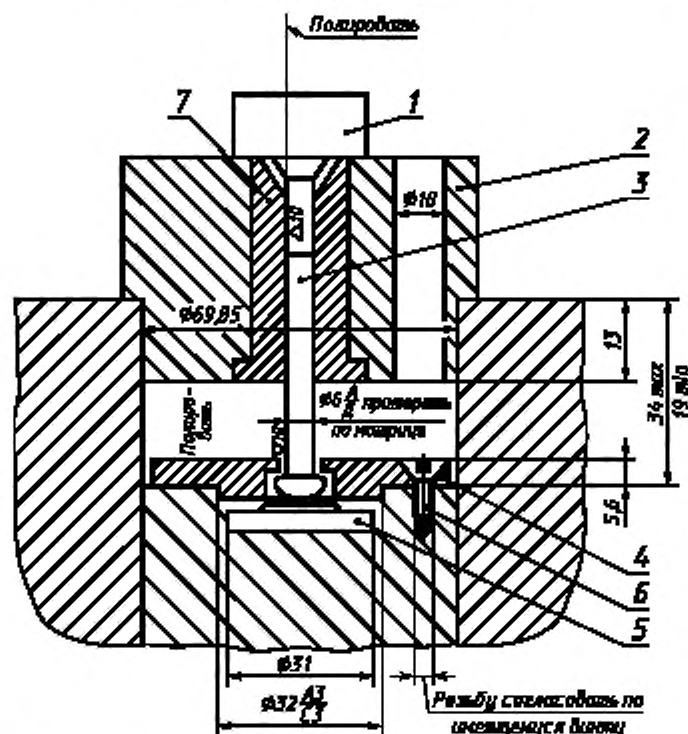
Комплект для прессования порошков
