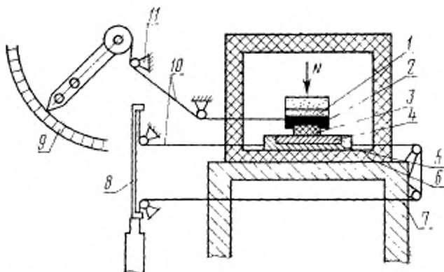
Установка по определению коэффициента трения
