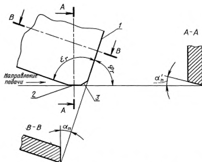
Т — главная режущая кромка; 2 — зачистная режущая фаска; 3 — переходная фаска
