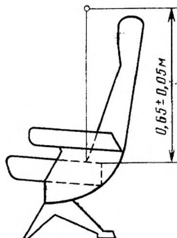
Расположение микро- фона на пассажирском кресле
