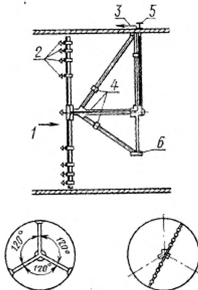
1—направление течения; 2—гидрометрические вертушки; 3—линия к хронографу; 4—держатель-треуго; 5—привод штанги; 6—опорная база треуго
