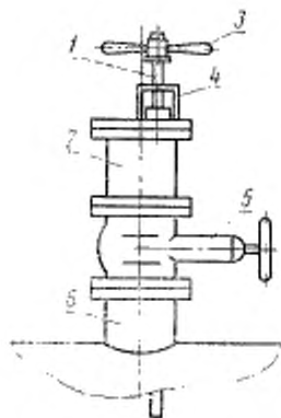
1—штатив-держатель средства измерений; 2—шлюзовая камера; 3—выравнивающий рычаг; 4—сальниковый ввод; 5—задвижка (затвор); 6—патрубок
