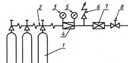
б) Рампа с 6 и менее баллонами
