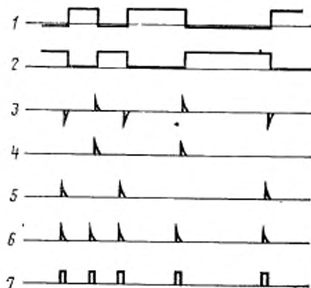
1—входной сигнал; 2—сигнал после формирователя; 3—сигнал на выходе дифференцирующей цепи; 4—неинвертируемые положительные импульсы; 5—сигнал на выходе инвертора; 6—сигнал на входе мультивибратора; 7—выходные импульсы
