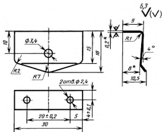
Зашелка
