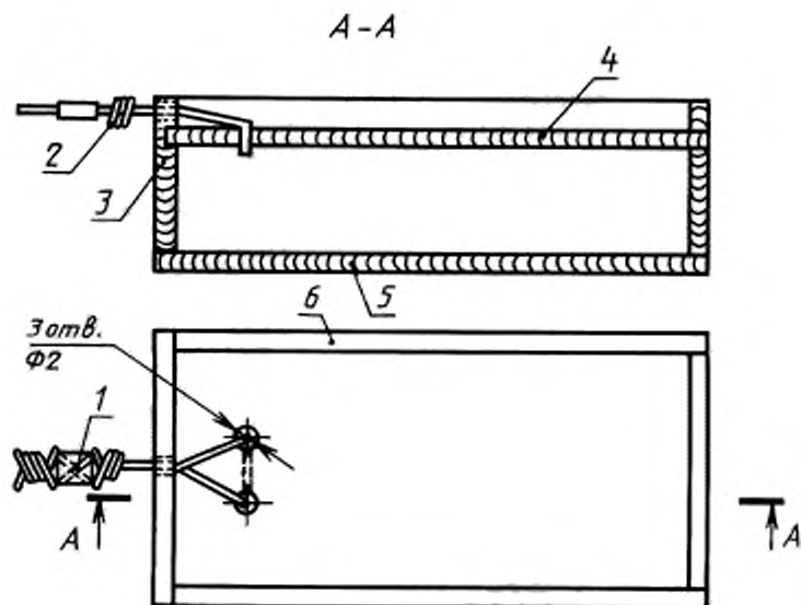
1 — пломба; 2 — проволока; 3 — торцовая стенка; 4 — крышка; 5 — дно; 6 — боковая стенка
