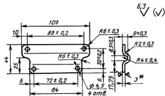
Накладка
