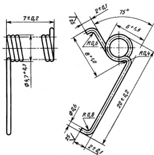
Пружина
