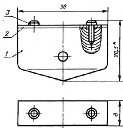
Зашелка
