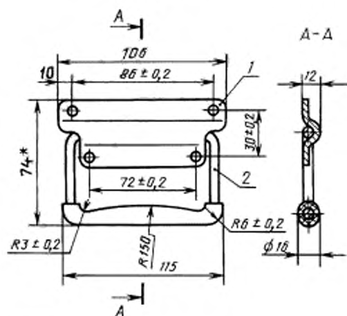
Ручка 4
