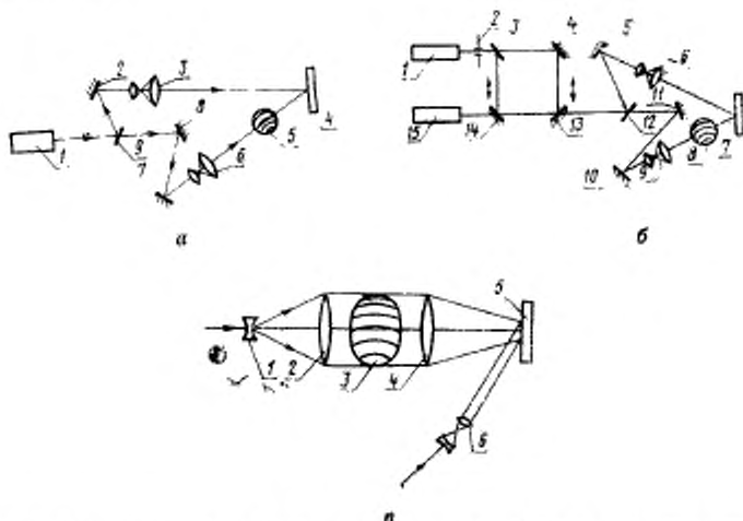
а—для стационарных объектов; б—для нестационарных объектов; в—участок схемы с большой апертурой сигмального пучка
