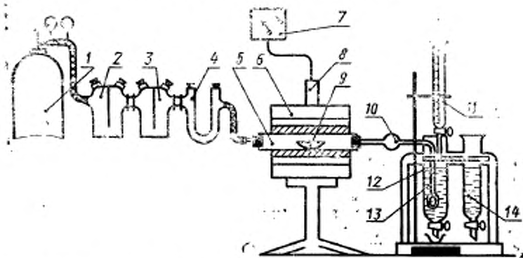
Установка для определения содержания серы
