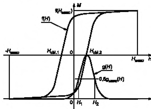
Рисунок 9 — Пример петли гистерезиса и ее дифференцированной кривой
