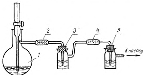
1—реакционная колба; 2, 4—трубки с сульфатом, пропитанным концентрированной серной кислотой; 3—приемник фтора, содержащий 15 см 3 дистиллированной воды; 5—приемник углекислого газа, содержащий 15 см 3 аммиачного раствора хлорида бария
