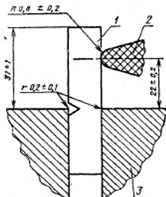
Схема испытания «перевернутого образца»
