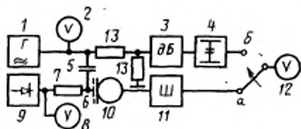
1—генератор; 2, 5—вольтметры; 3—магазин затуханий; 4—согласующее звено; 5—разделительный конденсатор; 6—электростатический возбудитель; 7—резистор; 8—источник поляризующего напряжения; 10—микрофон шумомера; 11—электрическая часть шумомера; 12—вольтметр или самописец; 13—делитель напряжения
