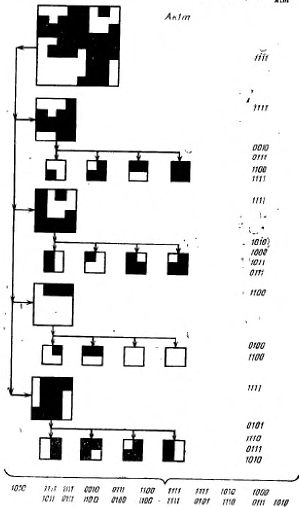
Пример кодирования не белого квадрата A_{k1m}
