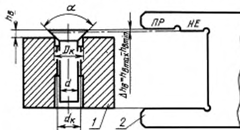
1 — тулза калибра; 2 — скоба калибра или индикатор
