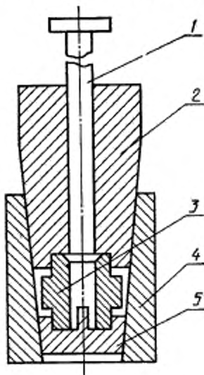
1 — пуансон; 2 — бункер; 3 — гнездо для тигля; 4 — обруч; 5 — пята
