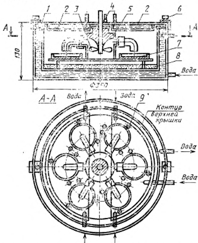
1—сосуд с двойными стенками; 2—крышка, состоящая из двух частей; 3—пропеллер; 4—термометр; 5—бронзовый подпятник; 6—винтовые зажимы; 7—бюксы; 8—насыщенный раствор сульфата калия; 9—шпигеты
