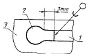
1 — печатный проводник; 2 — новая контактная площадка; 3 — материал основания Черт. 3
