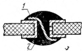
1 — перемычка; 2 — припой Черт. 2
