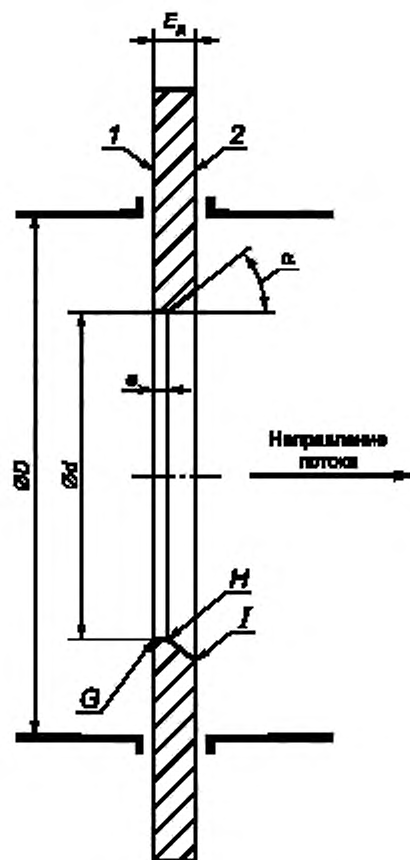
1 — входной торец диафрагмы; 2 — выходной торец диафрагмы
