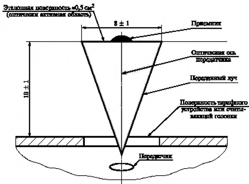
Рисунок 5 — Расположение передатчика при испытании
