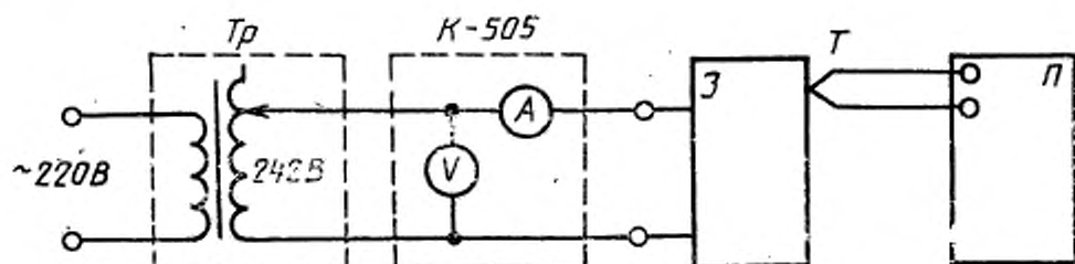
Тр — регулятор напряжения РНО; З — испытываемый звонок; П — автоматический потенциометр КСП-4; Т — термоэлектрический преобразователь ТХА
