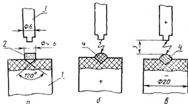
1 — графитовый электрод-подставка; 2 — таблетка пробы или стандартного образца; 3 — графитовый электрод; 4 — капля расплава. а — до экспонирования; б — при анодной подкисности таблетки; в — при катодной подкисности таблетки.
