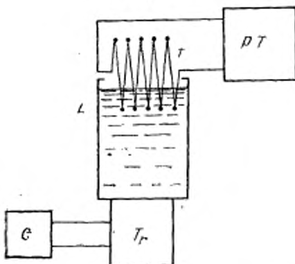
T_r — преобразователь; G — генератор возбуждения; L — ванна для воды (калориметр); T — термодатчик; PT — потенциометр
