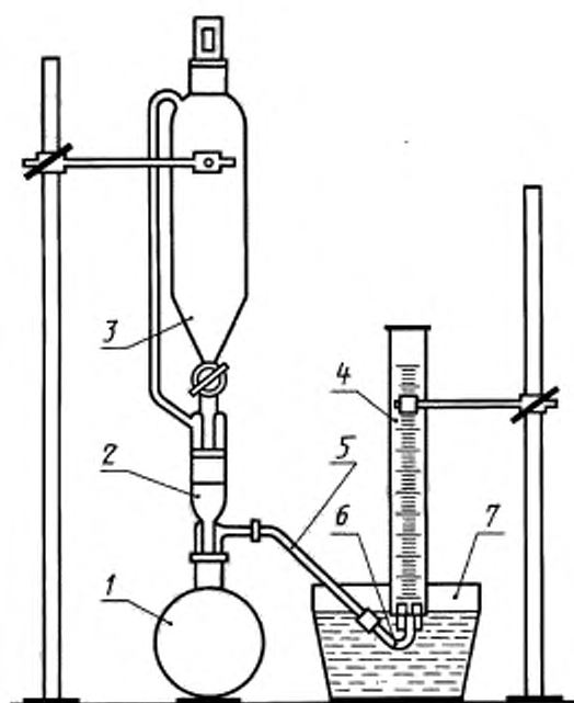
1 — колба лабораторная круглодонная; 2 — переход с одной горловиной и отводом; 3 — каплевая воронка; 4 — цилиндр мерный; 5 — трубка поливинилхлоридная; 6 — трубка стеклянная изогнутая; 7 — сосуд стеклянный четырехугольный
