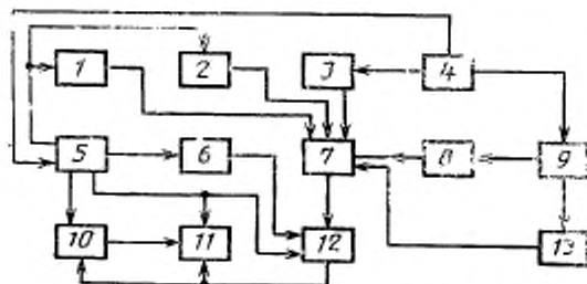
1—генератор гасящих импульсов; 2—блок разверток считывания; 3—источники питающих напряжений электродов трубки; 4—переключатель режимов работы трубки; 5—синхрогенератор считывания; 6—генератор калибровочных импульсов; 7—испытуемая трубка; 8—блок развертки записи; 9—синхрогенератор записи; 10—осциллограф с выделением строки; 11—видеоконтрольное устройство; 12—усилитель выходного сигнала; 13—генератор входного сигнала
