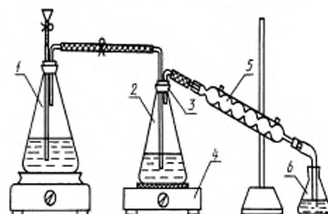
1 — колба-парообразователь с электроплиткой; 2 — перегонная колба; 3 — пробка с двумя отверстиями; 4 — электроплитка с асбестовой сеткой; 5 — стеклянный холодильник с алонжем; 6 — приемная колба
