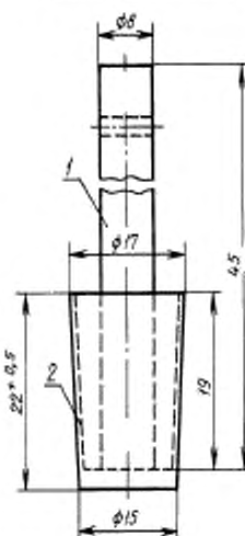
1 — стержень; 2 — тигель
