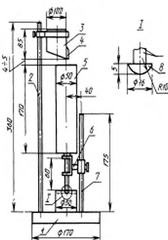
Прибор для определения прочности студня
