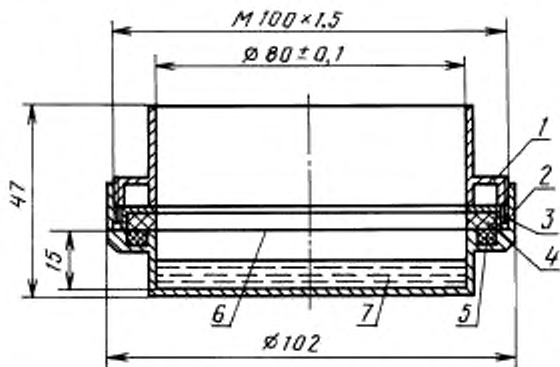
1 — специальная гайка; 2 — корпус; 3 — кольцо; 4, 5 — прокладки; 6 — образцы; 7 — вода
