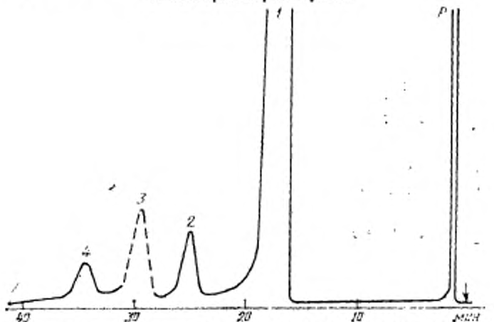
Типовая хроматограмма фенола
