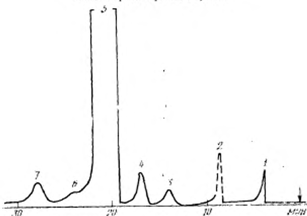
Типовая хроматограмма o -крезола
