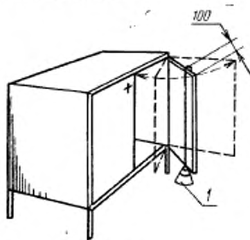
1 груз Черт. 2
