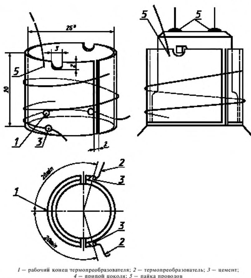
Рисунок 3 — Испытательный патрон для цоколей В22
