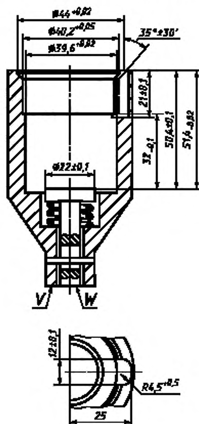
Рисунок А.4 — Калибр для проверки защиты от случайного прикосновения для ламп в резьбовых патронах с цоколем Е40
