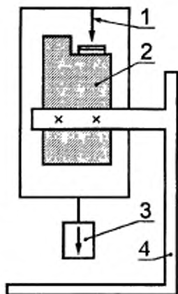
1 — направление усилия для искрообразования; 2 — корпус зажигалки, 3 — груз, 4 — штифт
