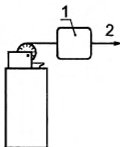
1 — динамометр; 2 — направление приложения усилия
