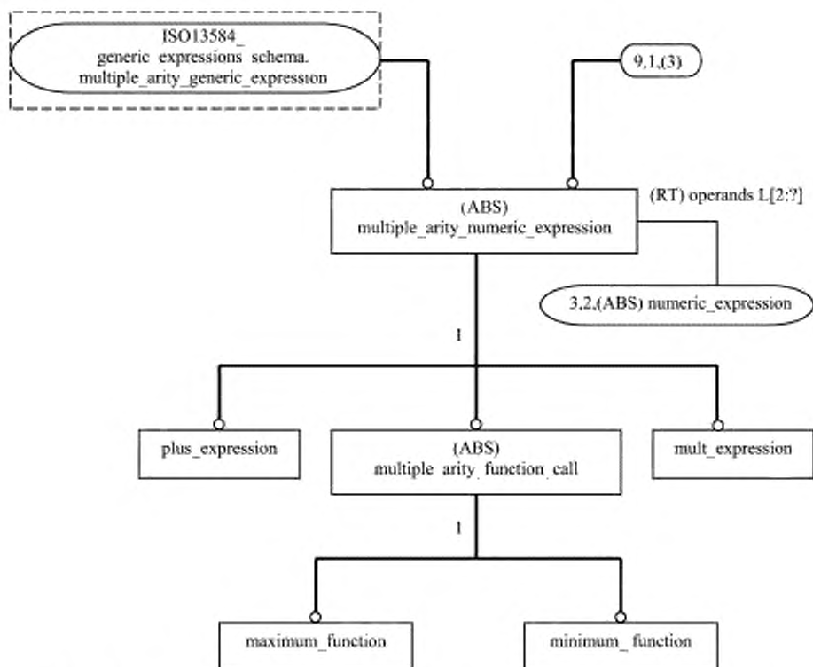
Рисунок С.10 — ISO13584_expressions_schema — EXPRESS-G диаграмма 9 из 12. Большая арифметика
