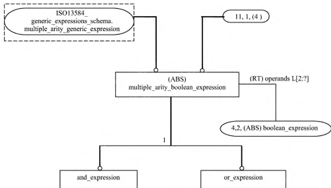
Рисунок С.12 — ISO13584_expressions_schema — EXPRESS-G диаграмма 11 из 12. Булевы выражения большой ариности
