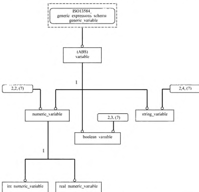
Рисунок С.3 — ISO13584_expressions_schema — EXPRESS-G диаграмма 2 из 12. Переменные
