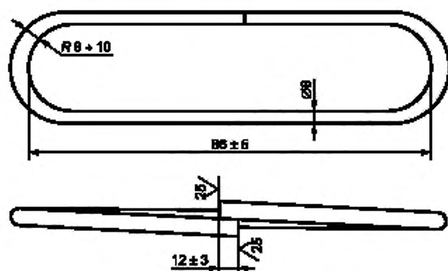
Рисунок 14 — Соединительное звено
