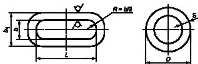
Рисунок 4 — Гильзовый сжим
