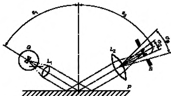
G — лампа; L 1 , L 2 — линзы; В — полевая диафрагма приемного устройства; Р — лакокрасочное покрытие; ε 1 — угол падения, ε 2 — угол отражения (ε 1 = ε 2 ); σ Г — апертурный угол приемной системы; σ В — апертурный угол изображения источника; I — изображение нити накала
