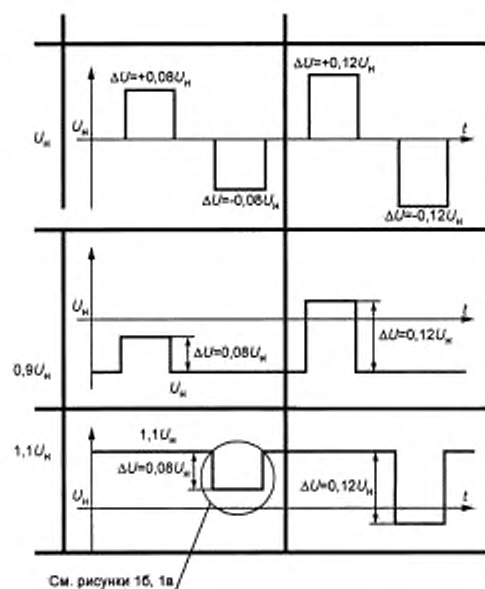
Рисунок 1а — Диаграмма колебаний напряжения
