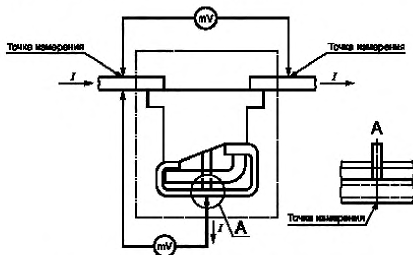
Рисунок 1 — Установка для испытания на падение напряжения
