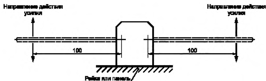
Рисунок 1 — Установка для испытания
