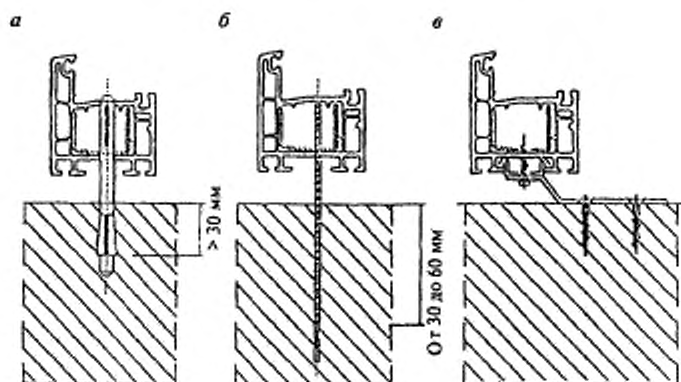
a — узел крепления монтажным дюбелем; b — узел крепления строительным шурупом; e — узел крепления при помощи анкерной пластины
