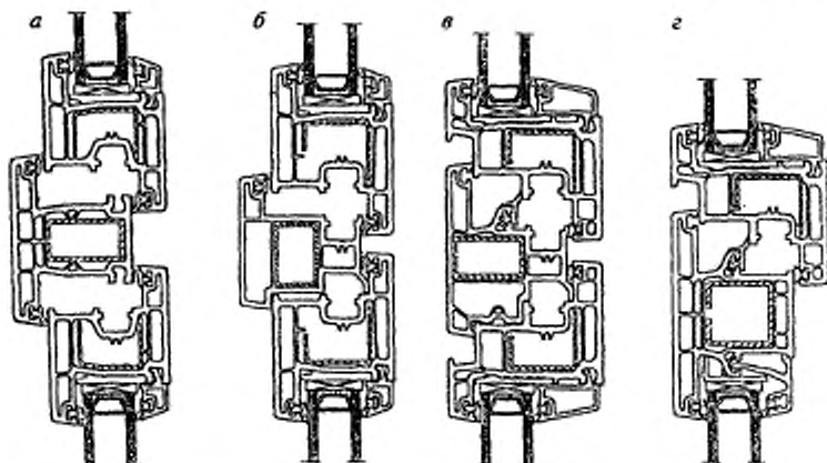
а — импостный притвор оконной системы с наружным и внутренним уплотнениями; б — штульповой (безимпостный) притвор оконной системы с наружным и внутренним уплотнениями; в — штульповой (безимпостный) притвор оконной системы со средним и внутренним уплотнениями; г — импостный притвор неоткрывающихся и открывающихся элементов оконной системы со средним и внутренним уплотнениями
