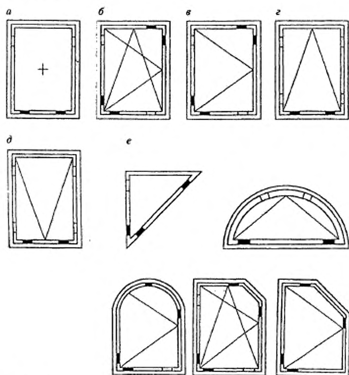
Виды открывания оконных блоков: a — неоткрывающиеся; б — поворотно-откидное; в — поворотное (распашное); г — откидное; д — подвесное; е — установка подкладок в фигурных оконных блоках
