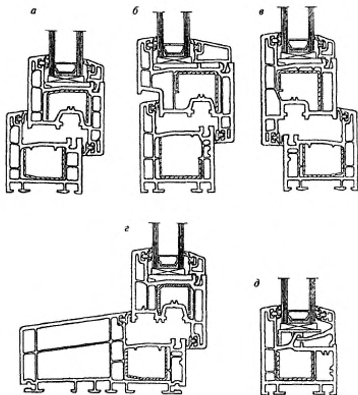
a — оконная система из трехкамерных профилей; б — оконная система с четырехкамерной створкой и трехкамерной коробкой (расположение наружных стенок створки и коробки в одной плоскости); в — оконная система из трехкамерных профилей (открывание наружу); г — оконная система из многокамерных профилей с расширенной коробкой; д — оконная система с остекленной коробкой
