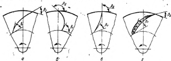
а — лопатки, загнутые назад ( \beta_2 < 90^\circ ); б — лопатки, загнутые вперед ( \beta_2 > 90^\circ ); в — лопатки, радиально оканчивающиеся ( \beta_1 = 90^\circ ); г — профильная лопатка
