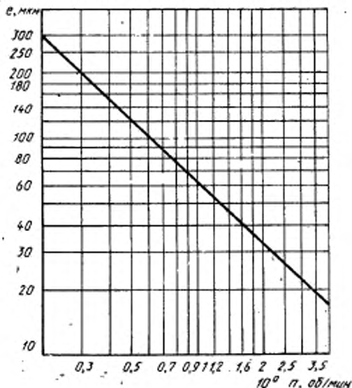
Допустимые удельные остаточные неуравновешенности рабочих колес вентиляторов
