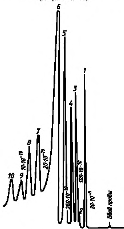
Типовая хроматограмма чистого 2-пиколина (альфа-пиколина)
