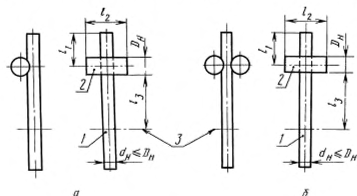
Форма и размеры образцов для испытания крестообразных соединений на срез
