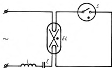
S — стартер; EL — люминесцентная лампа; L — C — индуктивно-емкостной балласт
