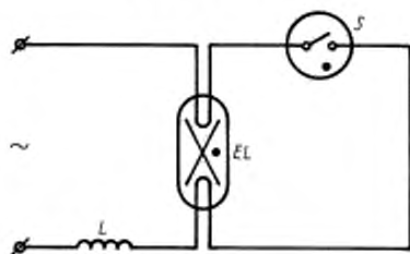
EL — люминесцентная лампа; S — стартер; L — индуктивный балласт
