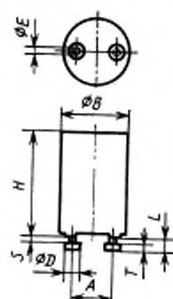
Размеры starters
