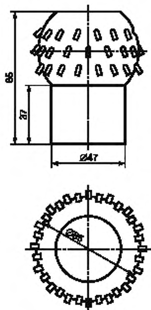
Защитный колпачок
