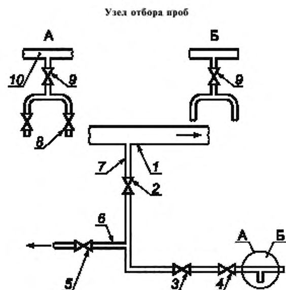
А — узел отбора проб с использованием пробоборной пробирки (черт. 5); Б — узел отбора проб с использованием пробоборной пробирки (черт. 4); 1 — трубопровод для сжиженного безводного аммиака; 2, 3, 8, 9 — вентили для подачи сжиженного безводного аммиака; 4 — вентиль тонкой регулировки; 5 — вентиль для сброса аммиака в дренажную систему; 6 — продувочная линия; 7, 10 — пробоборная линия
