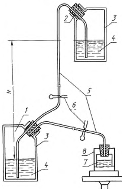
1 — сжатый воздух; 2 — пробка; 3 — канистра; 4 — вода; 5 — трубка; 6 — зажим; 7 — анализируемая проба; 8 — во- ронка фильтровальная
