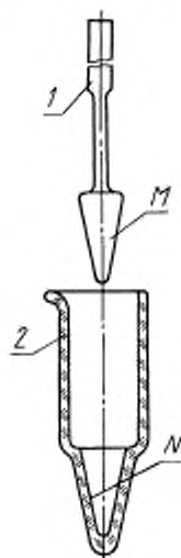
Схема гомогенизатора
